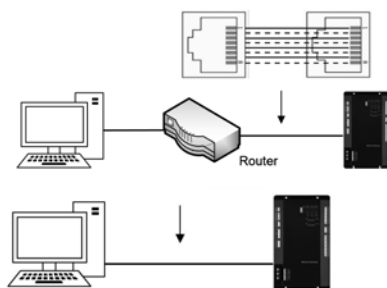
Schemat instalacji komunikacji bramki BACnet - komputer
