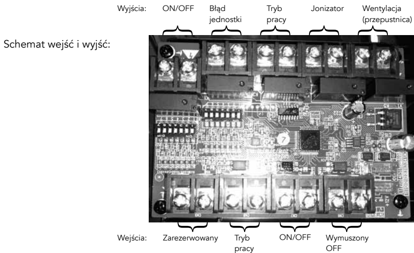
Schemat sygnałów modułu Dry Contact
