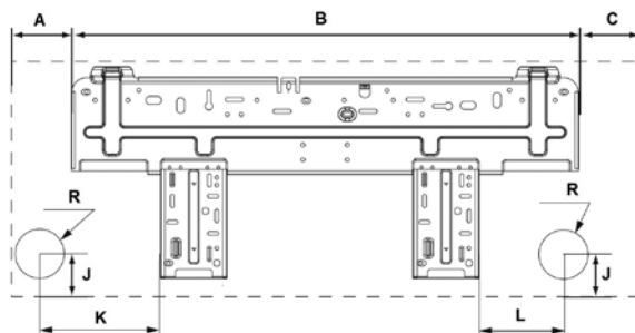
Blacha montażowa
